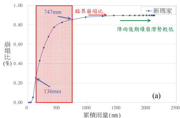
圖 12 高屏河流域新瑪家雨量站臨界雨量值訂定
