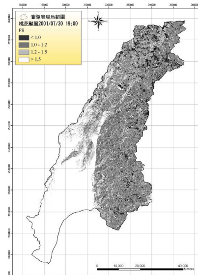
圖 9 率定結果與桃芝颱風山崩目錄之套疊比對
