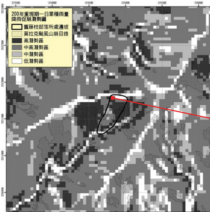
圖 15 藤枝地區降雨促崩潛勢分布圖 Fig.15 Landslide potential map in the Teng-Zhi area.
