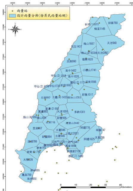
圖 11 高屏河流域 200 年重現期 24 小時累積雨量 (徐昇氏雨量站網)
